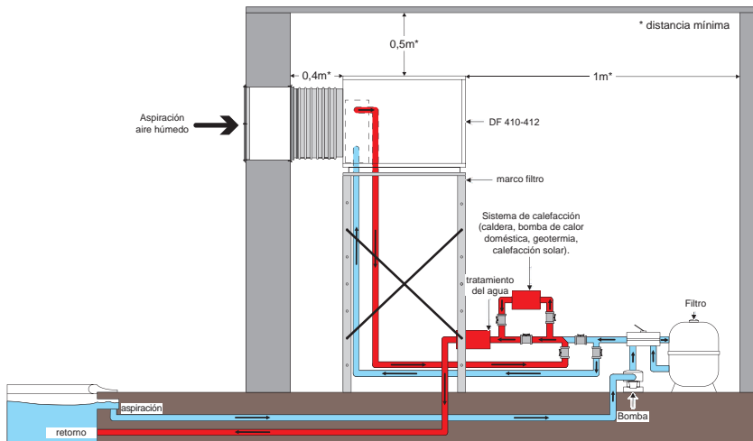
Ejemplo de instalación de un Sirocco Ambiente
